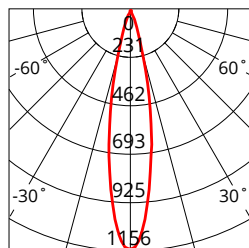
Unit: cd - C0/180 20.0deg - C90/270 19.4deg
