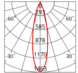
Unit: cd - C0/180 24.6deg - C90/270 24.5deg
