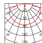
Unit: cd C0/180 153.4deg C90/270 154.1deg
