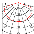
Unit: cd C0/180 145.2deg C90/270 151.4deg
