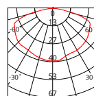
Unit: cd C0/180 150.7deg C90/270 149.9deg
